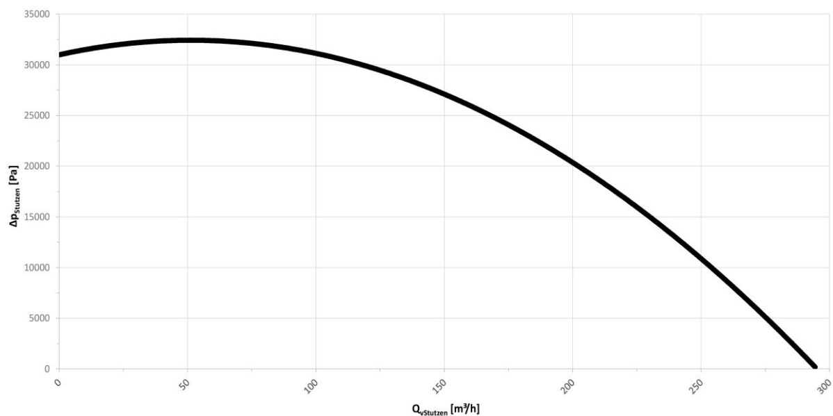
16. ábra: Jelleggörbe
